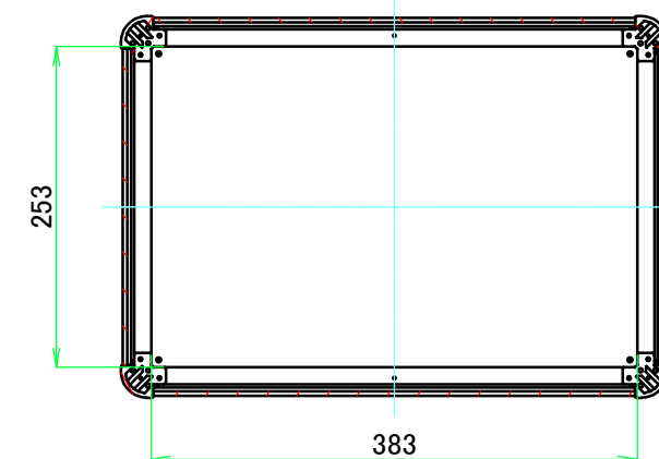
C-C ( 1 : 6.5 )
